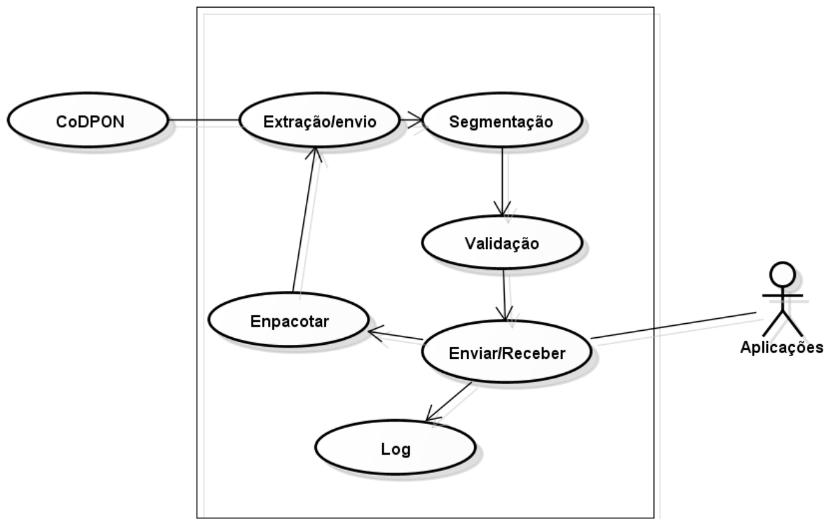
Figura 5. Diagrama de Representação da Interação CoDPON x Arquitetura x Aplicações.
